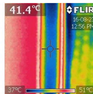
ネット下 屋根温度
