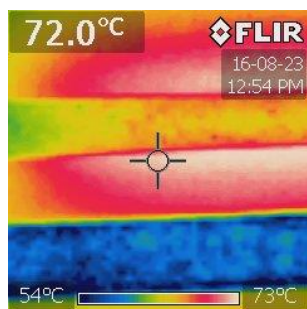
ネット無 屋根温度
